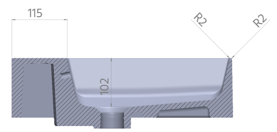
Sektion A-A
